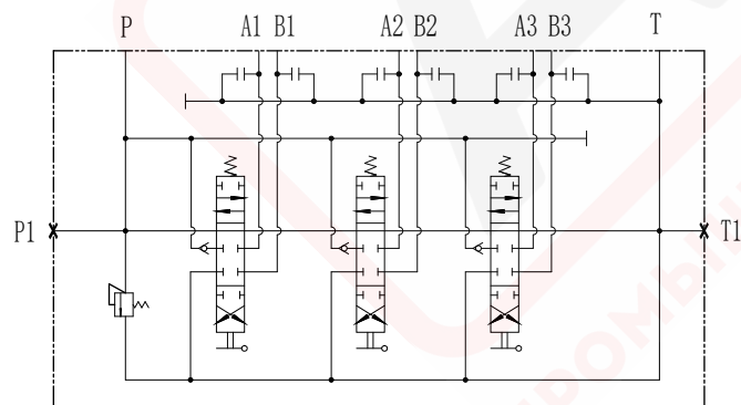
液压原理图
